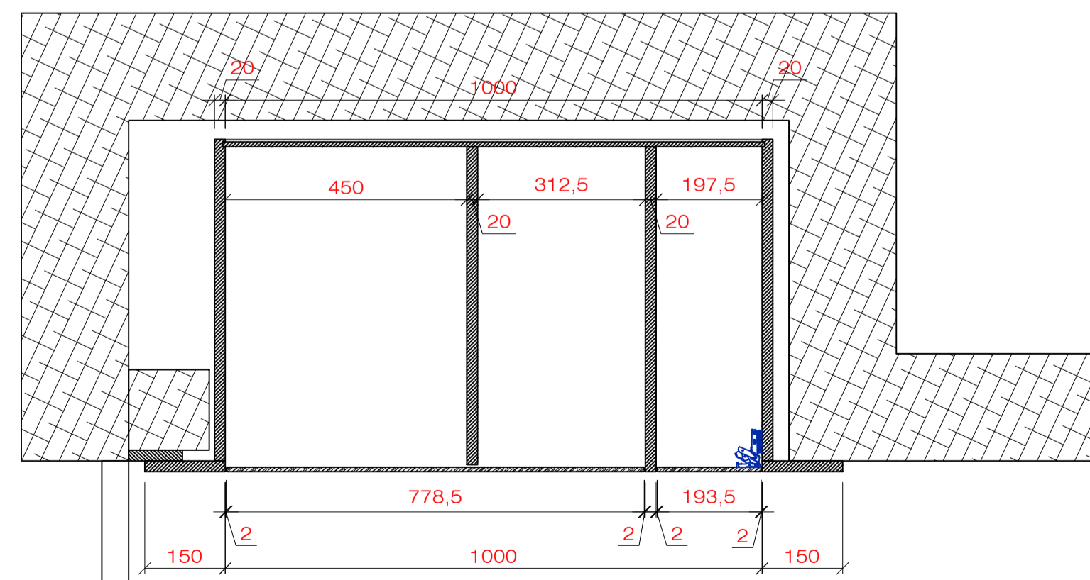
Sezione pianta "C-C" Scala 1:10
