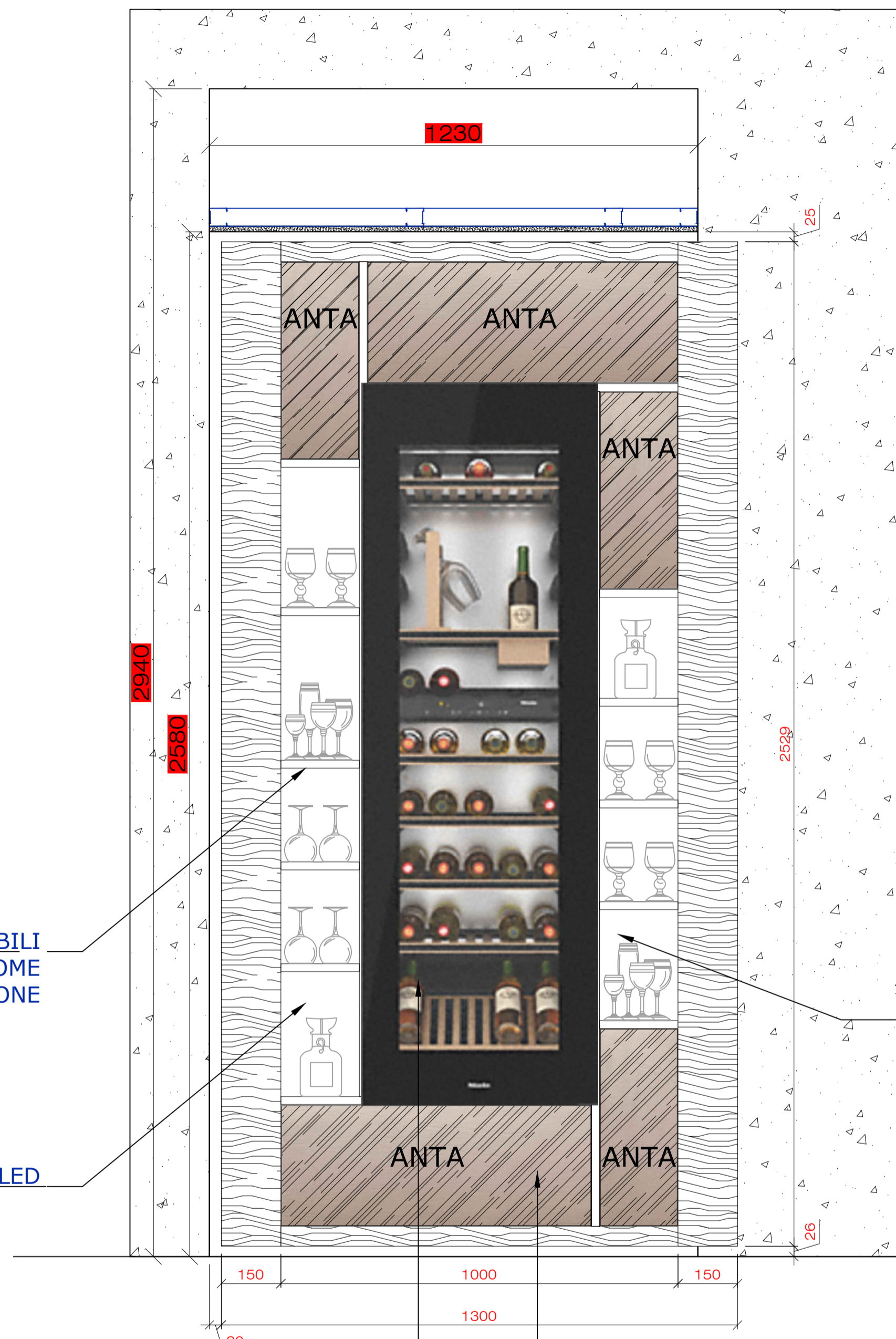
Vista frontale Scala 1:10
