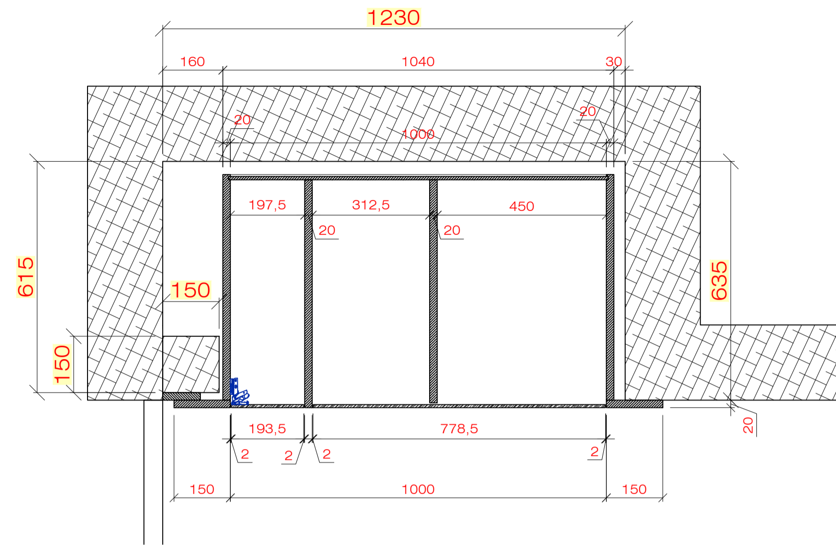
Sezione pianta "A-A" Scala 1:10
