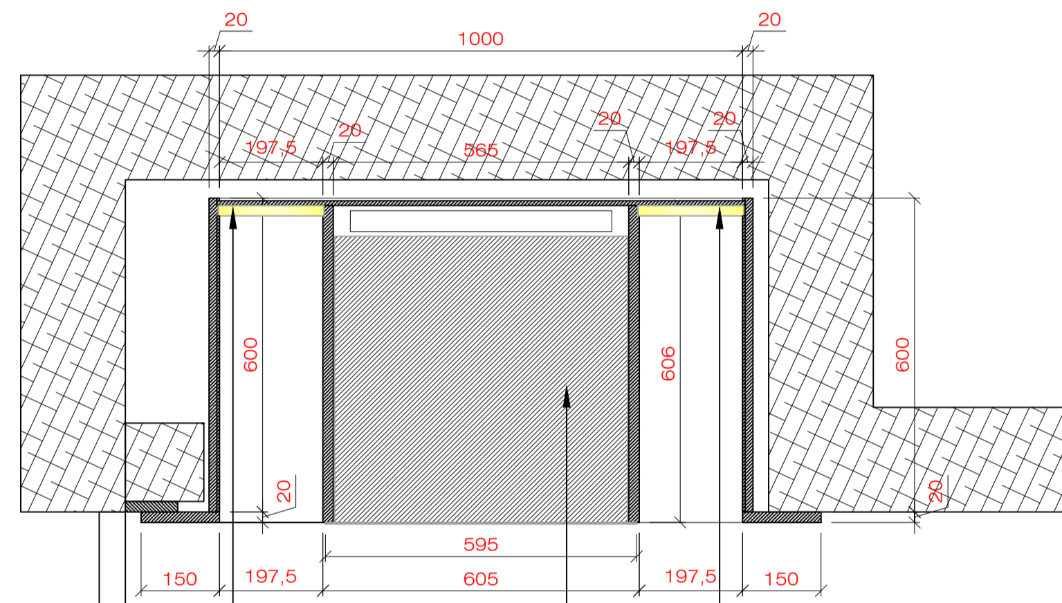
Sezione pianta "B-B" Scala 1:10
