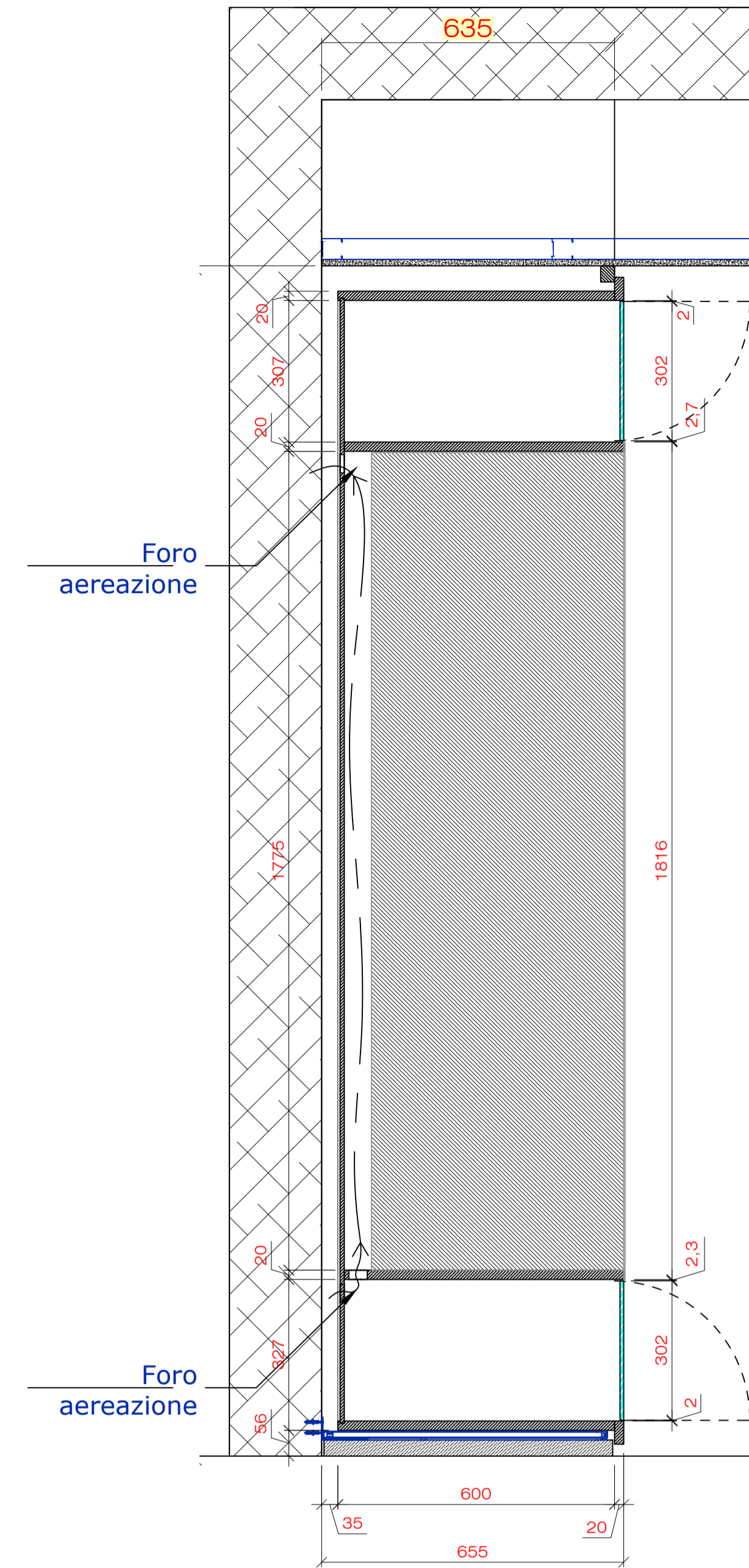
Sezione pianta "E-E" Scala 1:10
