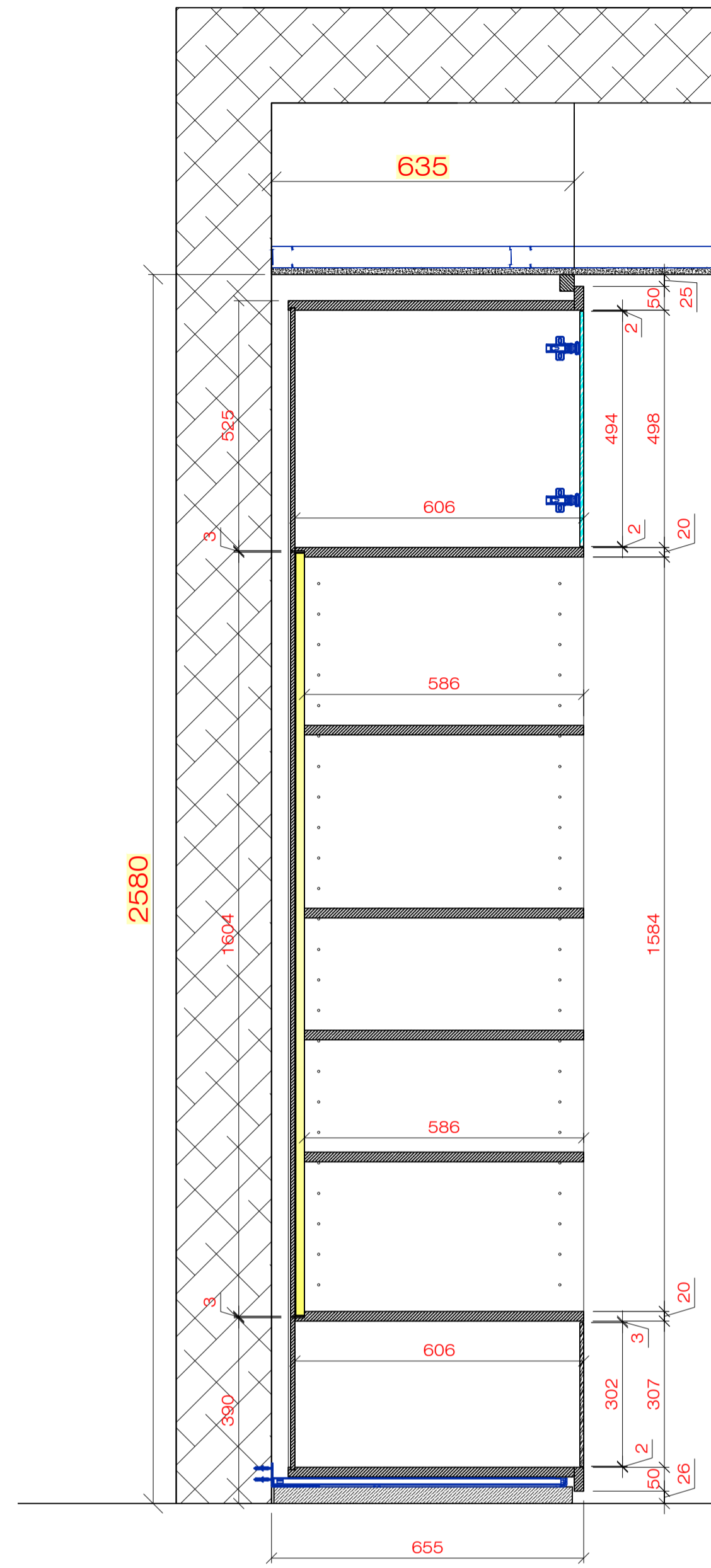
Sezione pianta "D-D" Scala 1:10
